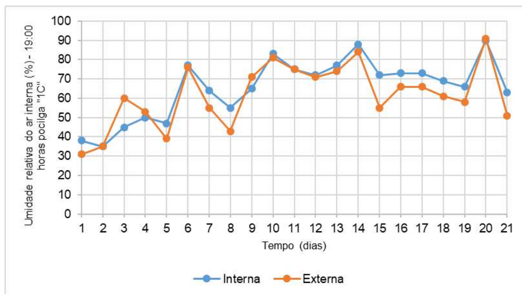
Figura 94 - Umidade relativa do ar interna x umidade relativa do ar externa do ambiente às 19:00 horas na pocilga "1C".
